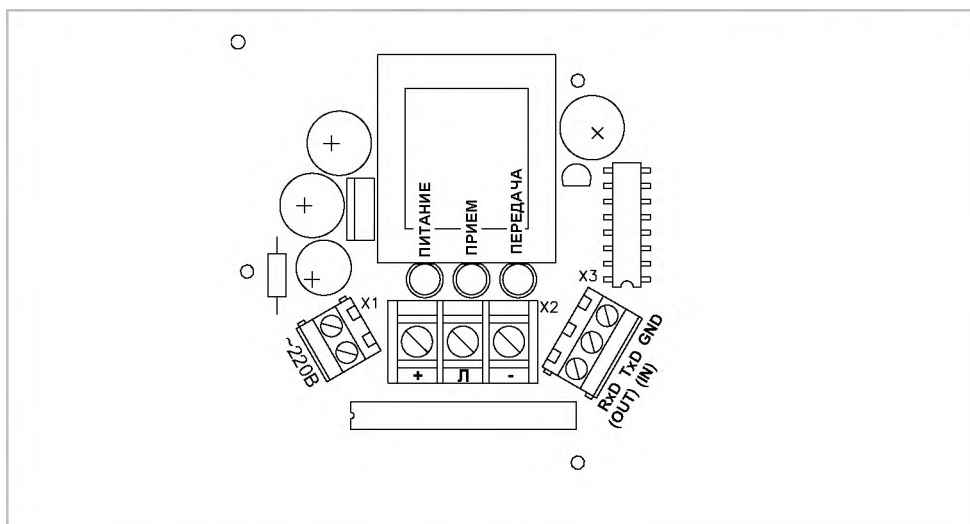
Рис.3. Внешний вид платы. Назначение контактов и индикаторов.
