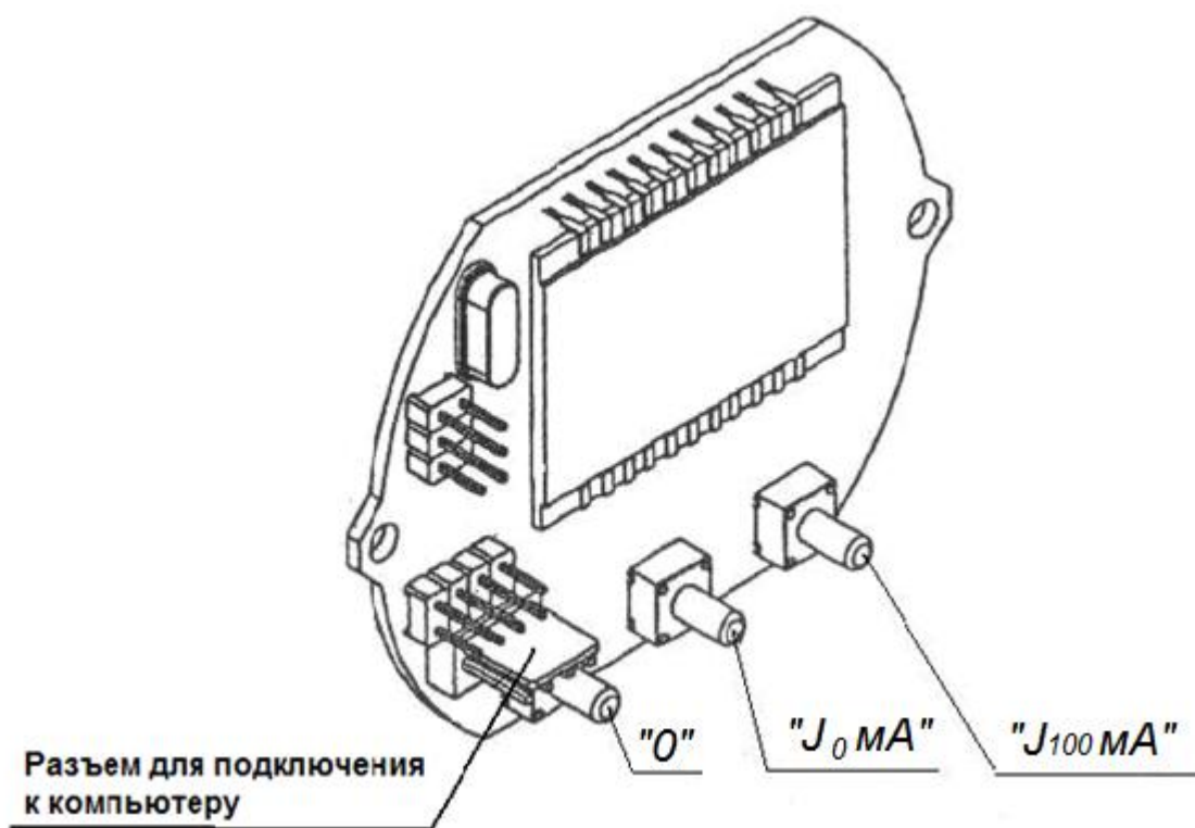
Рисунок 3 - Внешний вид платы электронного преобразователя
