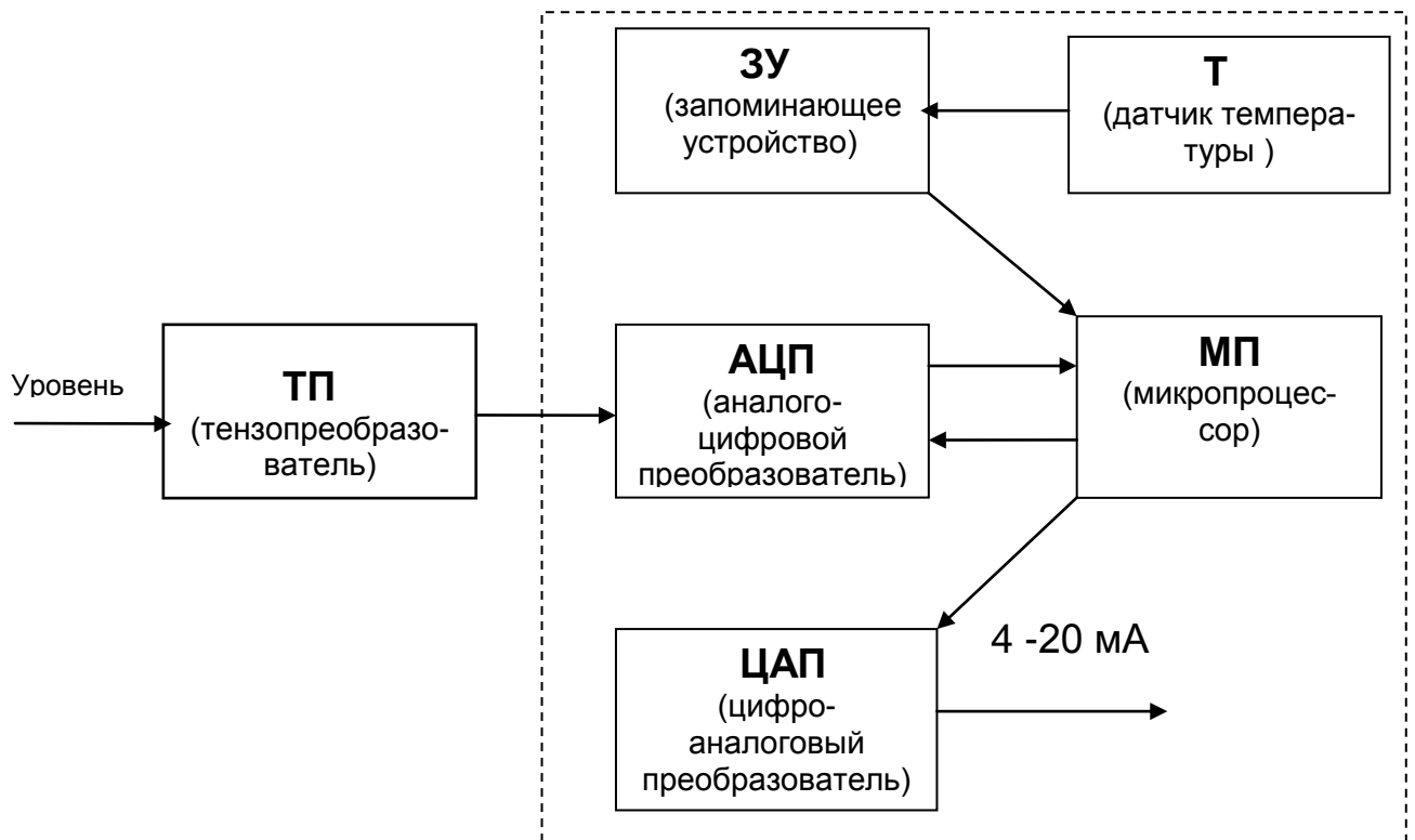
Рисунок 2 – Блок –схема преобразователя электронного
