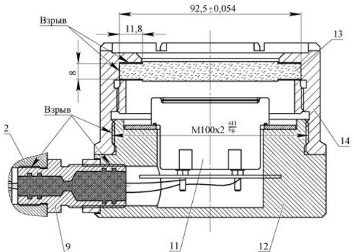
Е - Е (2:1)
