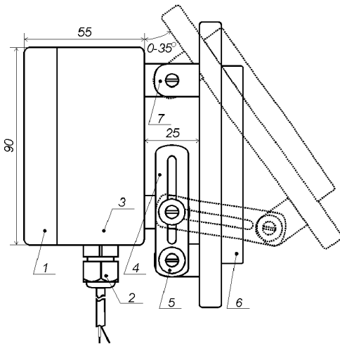
Рис. 5. Конструкция генератора ППМ-02РГ и детектора ППМ-02РД.
