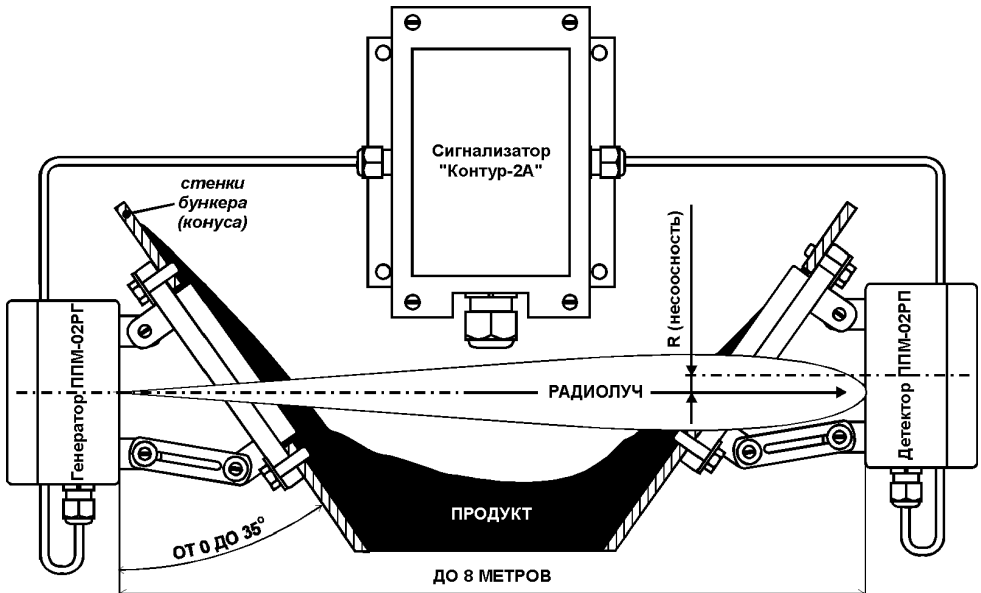
Рис. 1. Принцип действия датчика РСУ-1РА.
