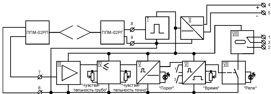
Рис. 2. Структурная схема датчика РСУ-1РА.
