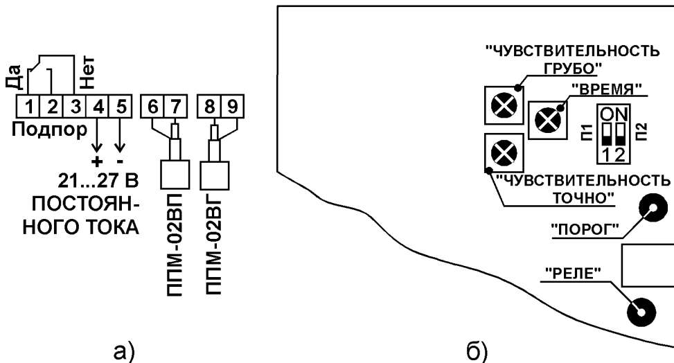
Рис. 6. Схема подключения и органы регулировки датчика PCSU-1P-2A.
