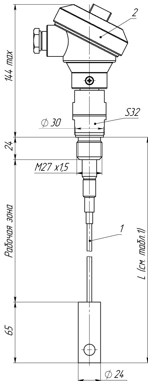
Рис. В.8 – Преобразователь первичный ПП-294, ПП-294И
