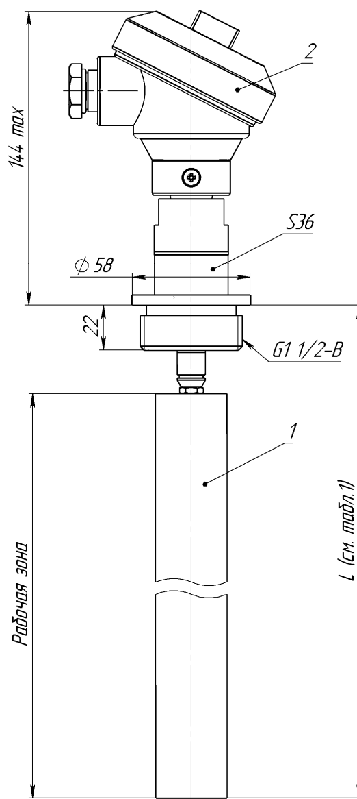
Рис. В.2 – Преобразователь первичный ПП-216, ПП-216И
