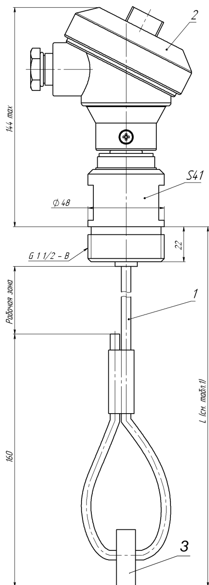
Рис. В.7 – Преобразователи первичные ПП-292, ПП-292И, ПП-296, ПП-296И
