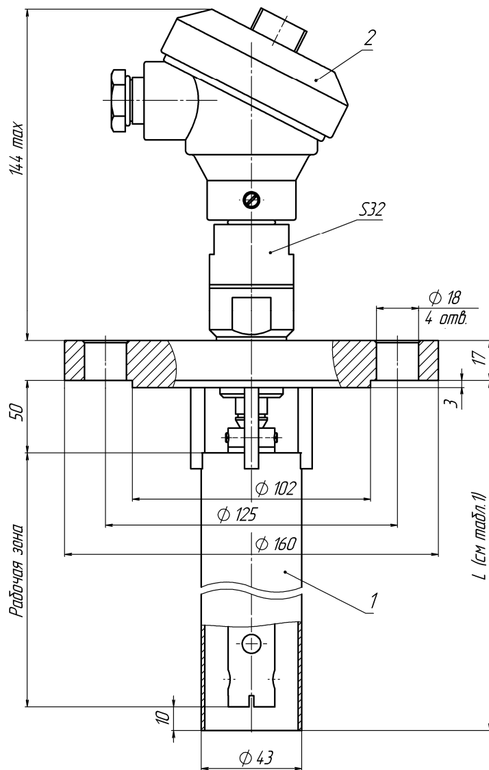
Рис. В.6 – Преобразователь первичный ПП-282, ПП-282И
