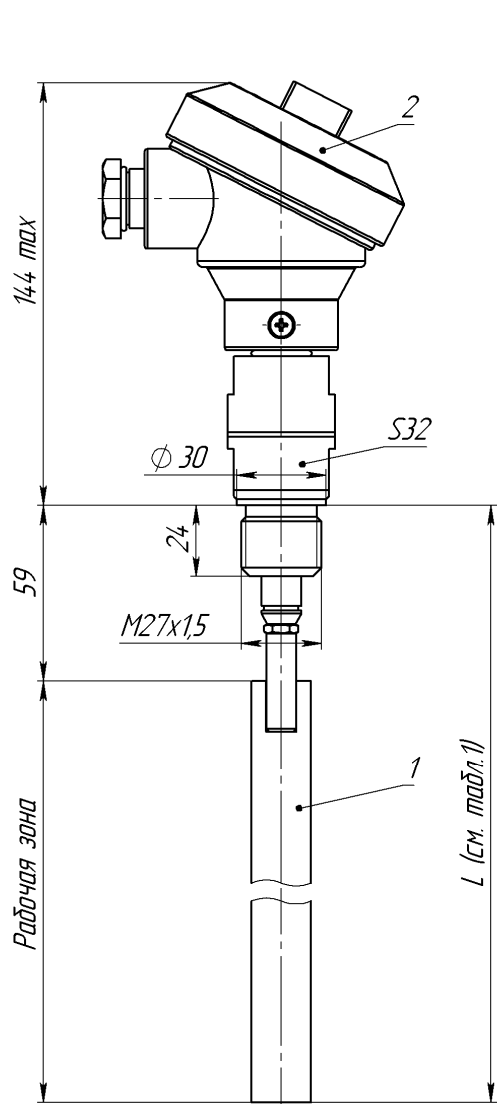
Рис. В.1 – Преобразователь первичный ПП-212, ПП-212И
