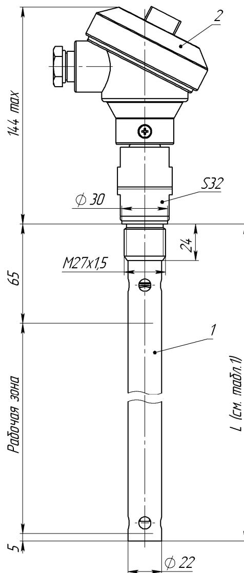
Рис. В.4 – Преобразователь первичный ПП-264, ПП-264И
