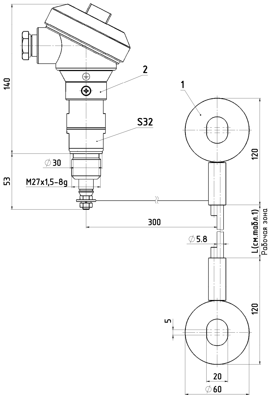
Рис. В.9 – Преобразователь первичный ПП-295
