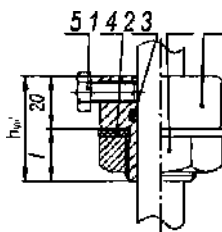
1 - Прокладка; 2 - Гайка; 3 - Штуцер; 4 - Кольцо
