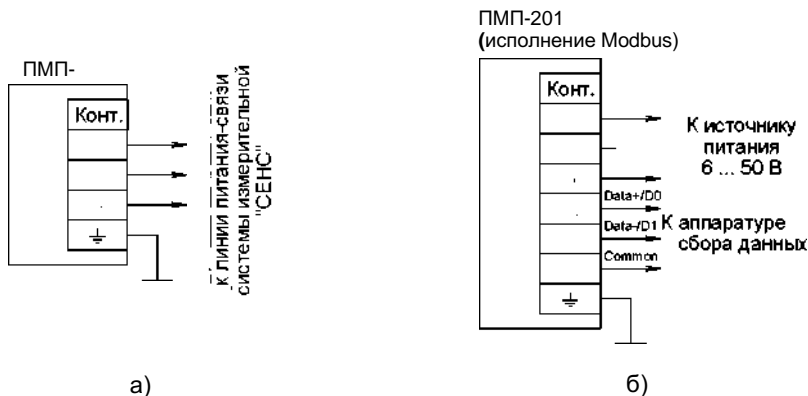
Рисунок 14 - Схема подключения:
