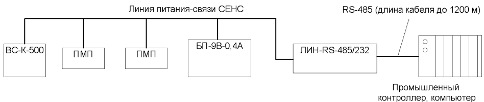
Рисунок 1 - Вариант применения адаптера совместно с устройствами СЕНС
