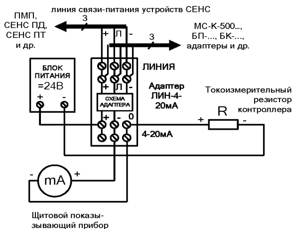
Рисунок 2. Схемы подключения:
