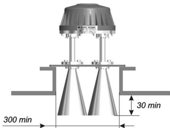
Рисунок 8 – Пример установки прибора исполнений БАРС 352И.22, БАРС 352И.26, БАРС 352И.30, БАРС 352И.34
