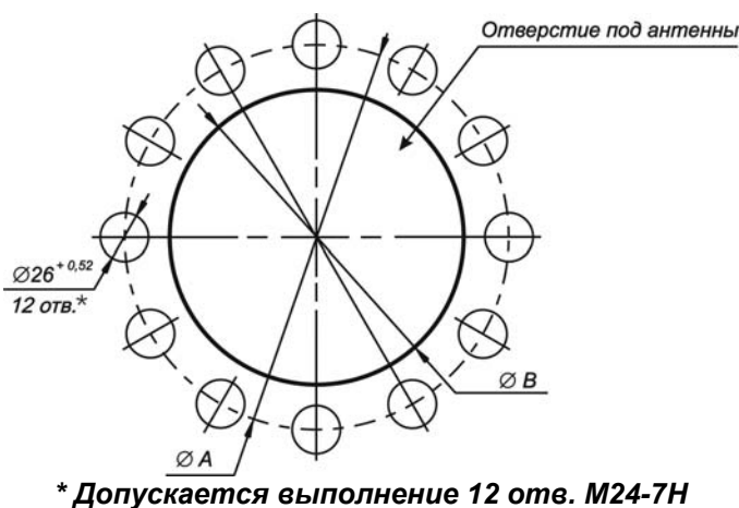
Рисунок 4 – Разметка для крепления приборов исполнений БАРС 352И.32, БАРС 352И.34
