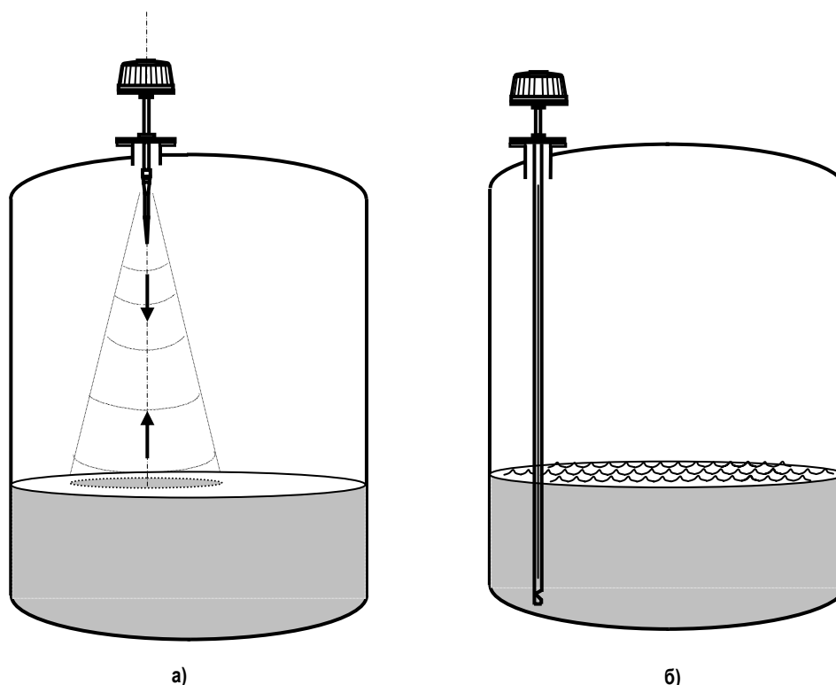
Рисунок 9 - Positionирование прибора на резервуаре с узким патрубком:
